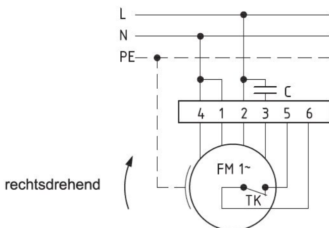
Anschlußplan 0.11-1 r.
