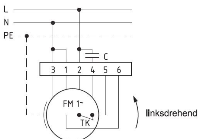
Anschlußplan 0.11-1 l.
