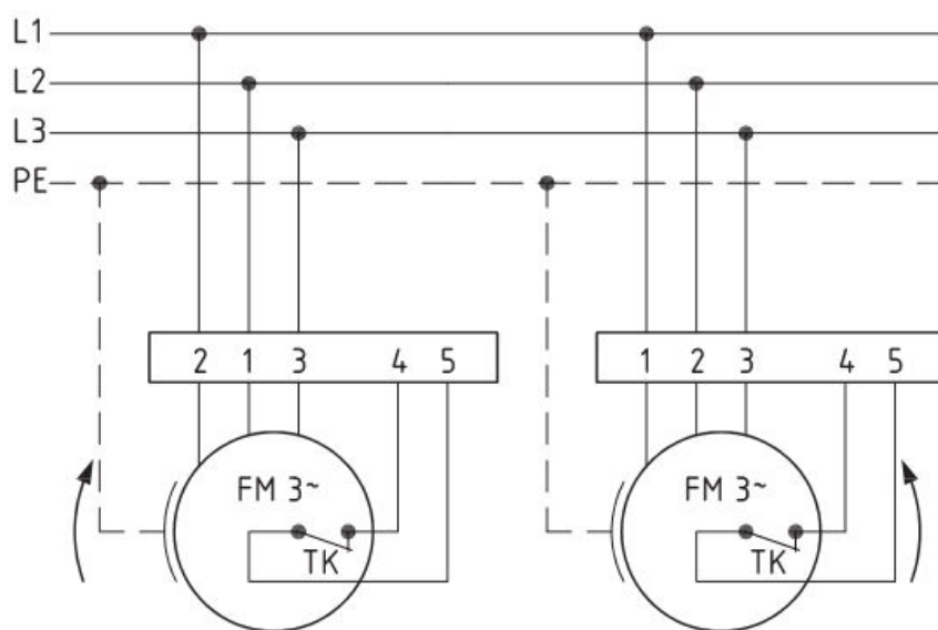
Anschlußplan 0.16-1 / 0.16a-1
