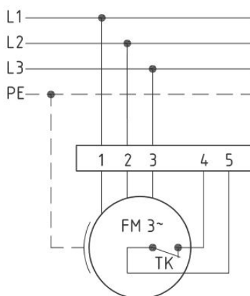
Anschlußplan 0.13-2 l.
