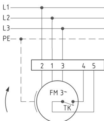
Anschlußplan 0.13-2 r.
