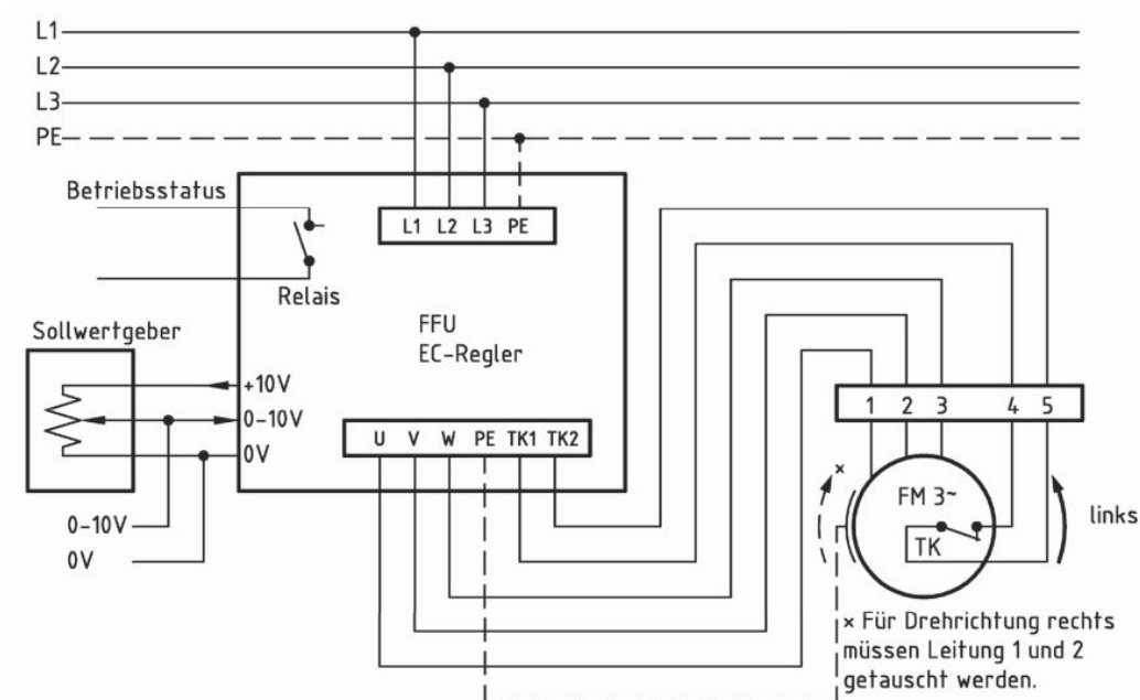
Anschlußplan* FFU-EC 400
