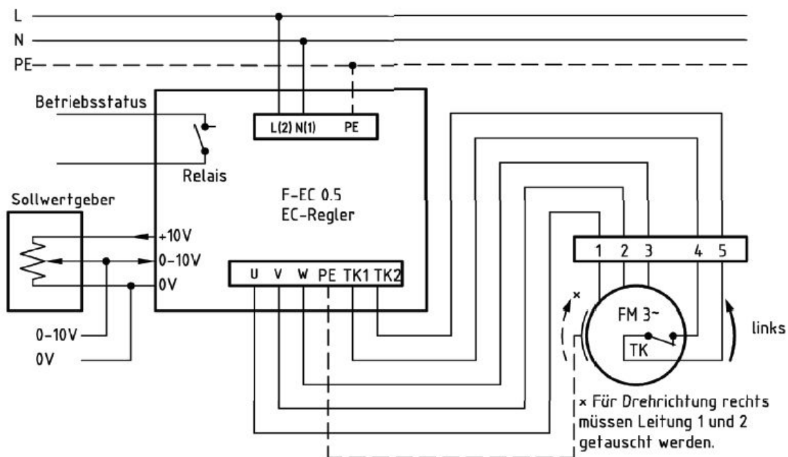
Anschlußplan* F-EC 0.5
