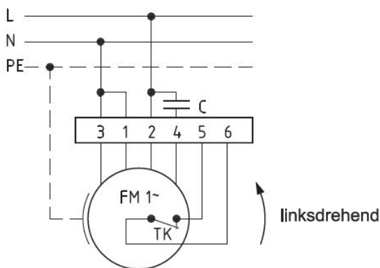
Anschlußplan 0.11-1 l.
