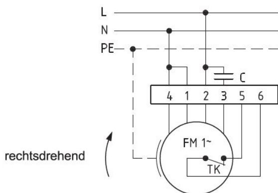
Anschlußplan 0.11-1 r.
