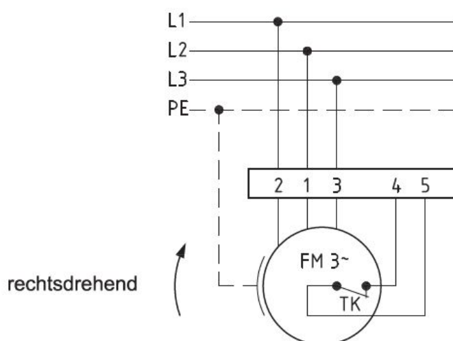
Anschlußplan 0.13-2 r.
