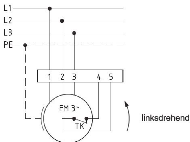
Anschlußplan 0.13-2 l.
