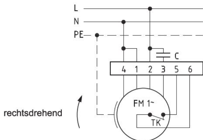
Anschlußplan 0.11-1 r.
