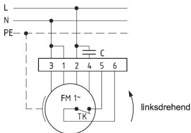
Anschlußplan 0.11-1 l.
