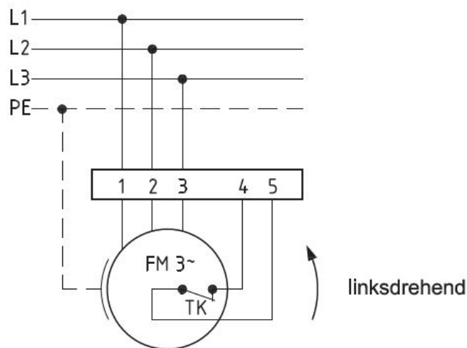
Anschlußplan 0.13-2 l.
