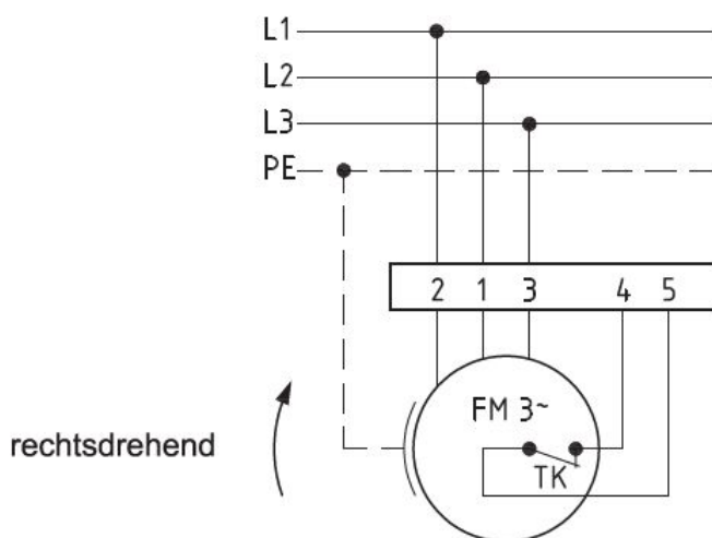
Anschlußplan 0.13-2 r.
