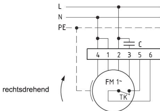
Anschlußplan 0.11-1 r.
