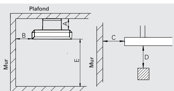
Fig. 1 : positionnement vertical.
