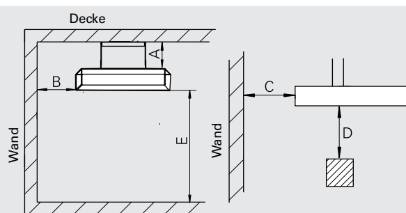
Abb. 1: Vertikale Ausrichtung.
