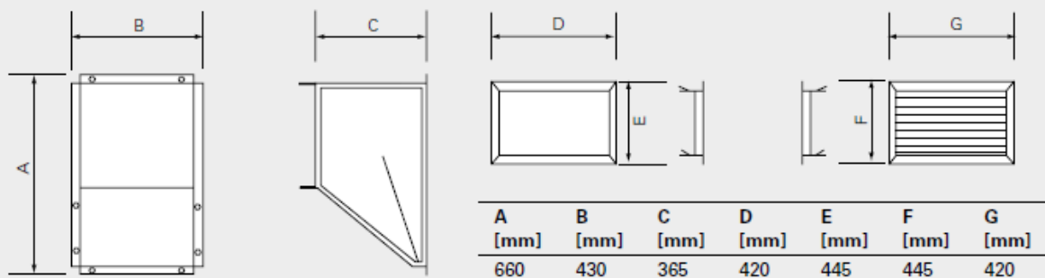
Mischluftkasten (Zubehör)
