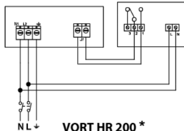
VORT HR 200 *
