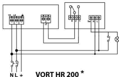
VORT HR 200 *
