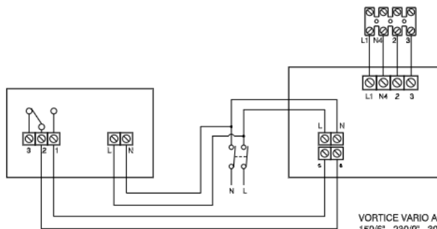
VORTICE VARIO AR - ARI 150/6" - 230/9" - 300/12"
