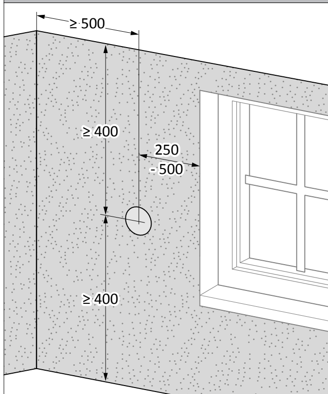
Abstand Kernloch (Laibungskanal)
