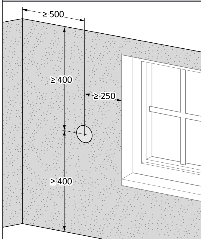
Abstand Kernloch (Wetterschutz Kunststoff, Wetterschutzhaube)
