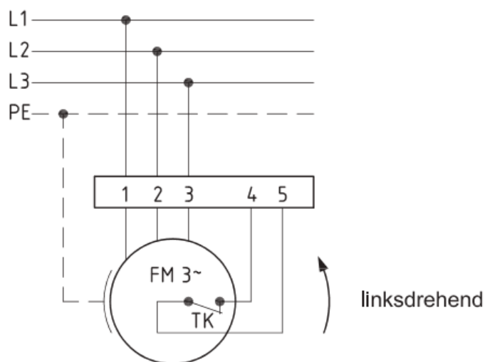
Anschlußplan 0.13-2 I.
